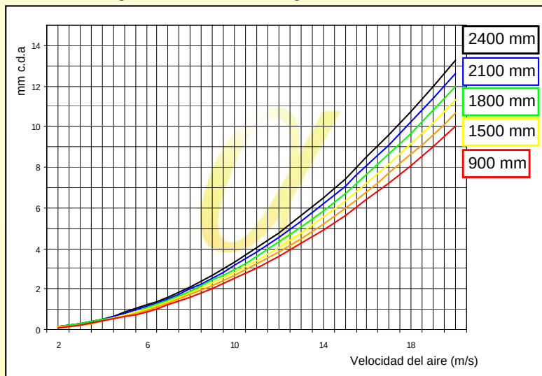
Pérdida de carga en función de la longitud
